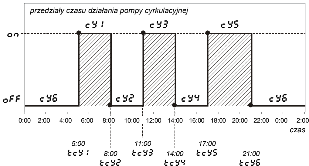
Rys. 24. Przykładowy program działania pompy cyrkulacyjnej.
