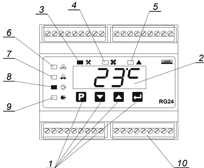
Rys. 5. Wygląd płyty czołowej regulatora.
