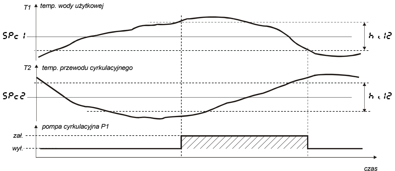
Rys. 22. Sposób działania pompy cyrkulacyjnej w trybie 3.
