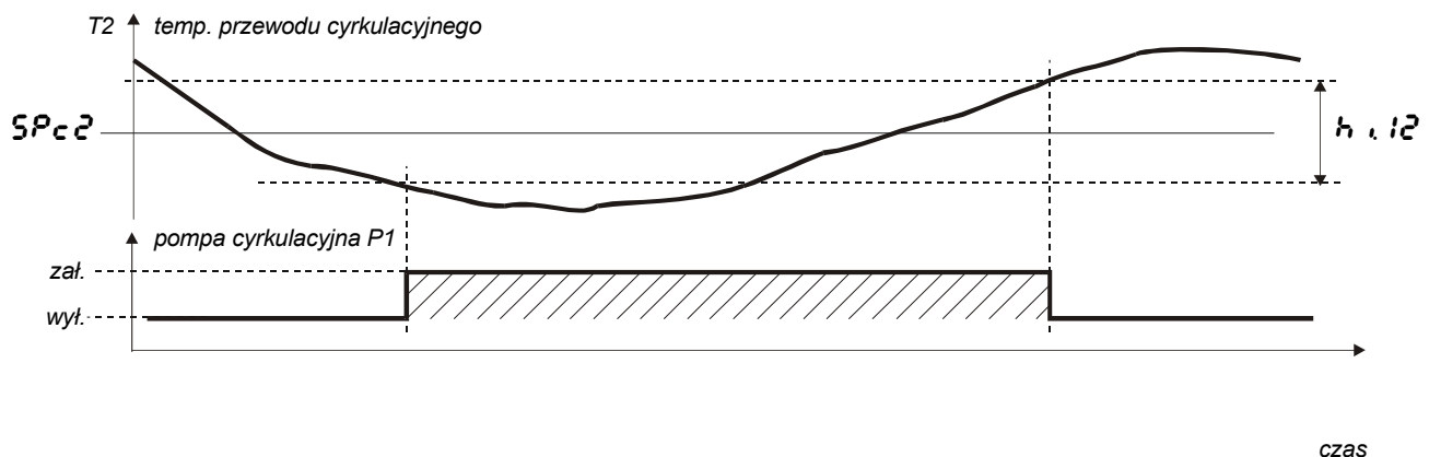
Rys. 21. Sposób działania pompy cyrkulacyjnej w trybie 2.
