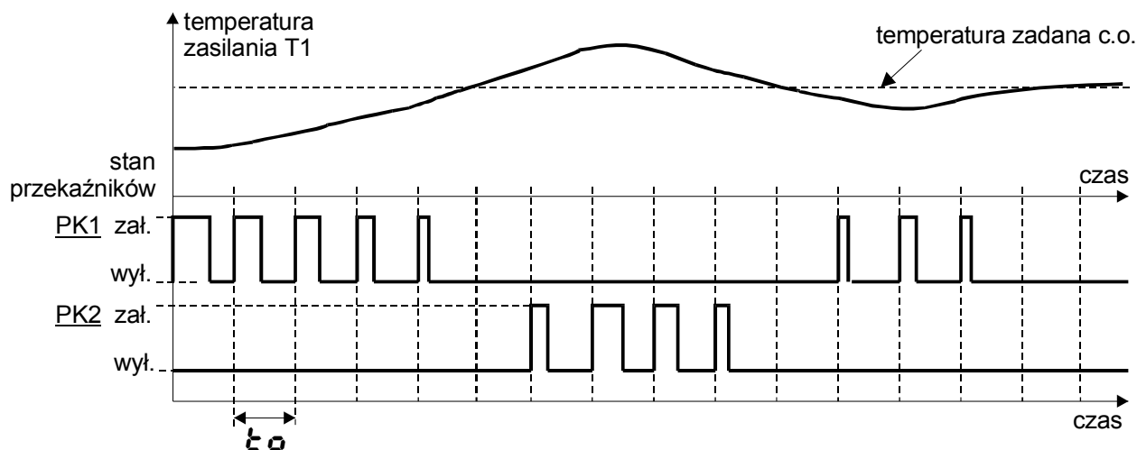
Rys. 10. Sterowanie napędem zaworu podczas regulacji trójstawnej krokowej PID.
