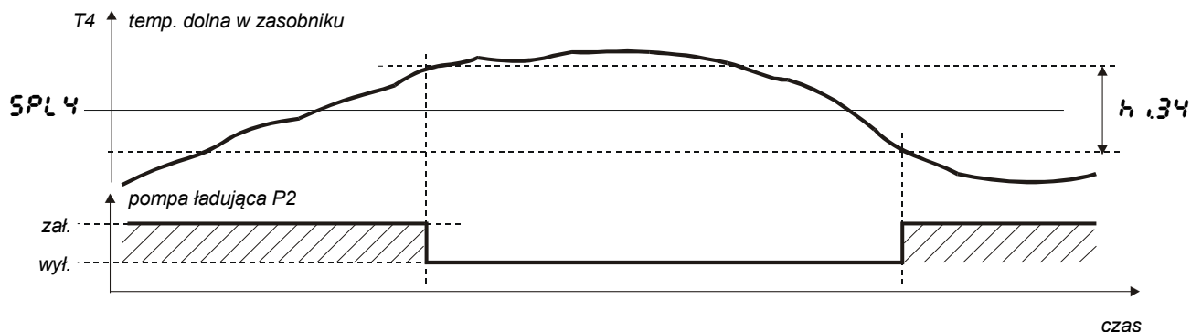
Rys. 29. Działanie pompy ładującej ze sprawnym tylko czujnikiem T4.
